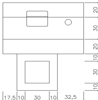
VISTA SUPERIOR EM PLANTA
