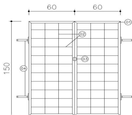
DETALHE - PORTÃO
