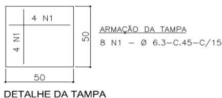
DETALHE DA TAMPA
