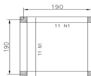
LAJE - ARMAÇÃO
