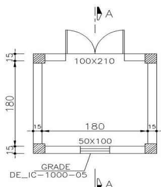
PLANTA BAIXA
